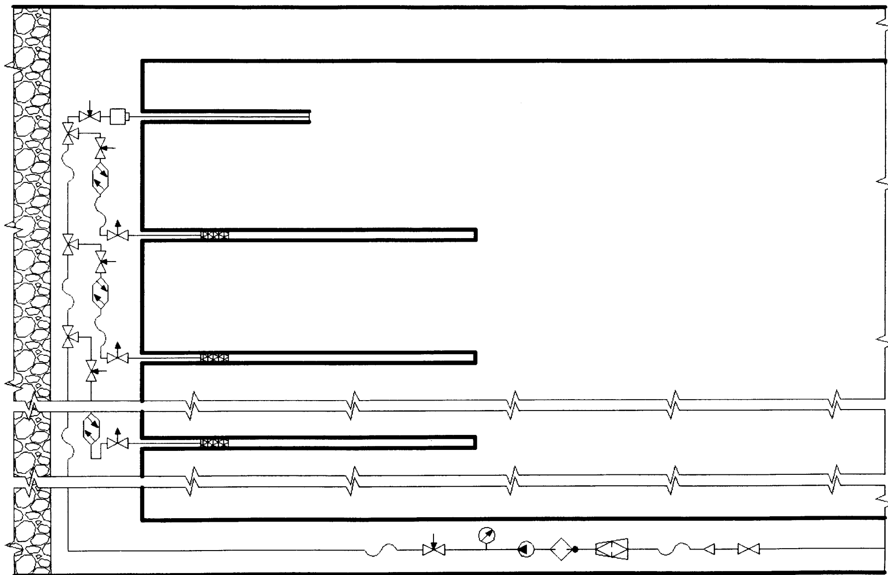
Рис. 3. Технологическая схема нагнетания жидкости в угольный пласт насосной установкой через скважины, пробуренные из очистного забоя (схема 3)
