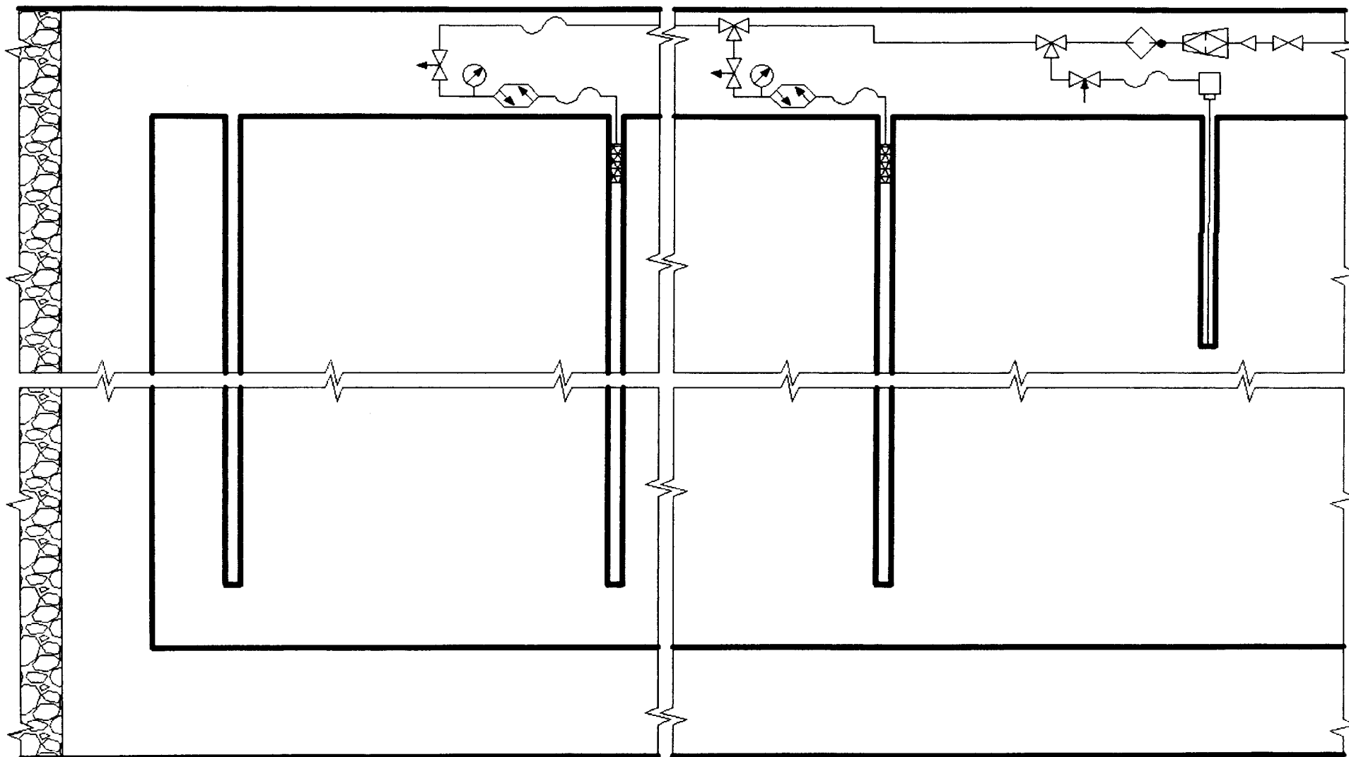
Рис. 4. Технологическая схема нагнетания жидкости в угольный пласт из противопожарно-оросительного трубопровода через скважины, пробуренные из подготовительной горной выработки (схема 4)
