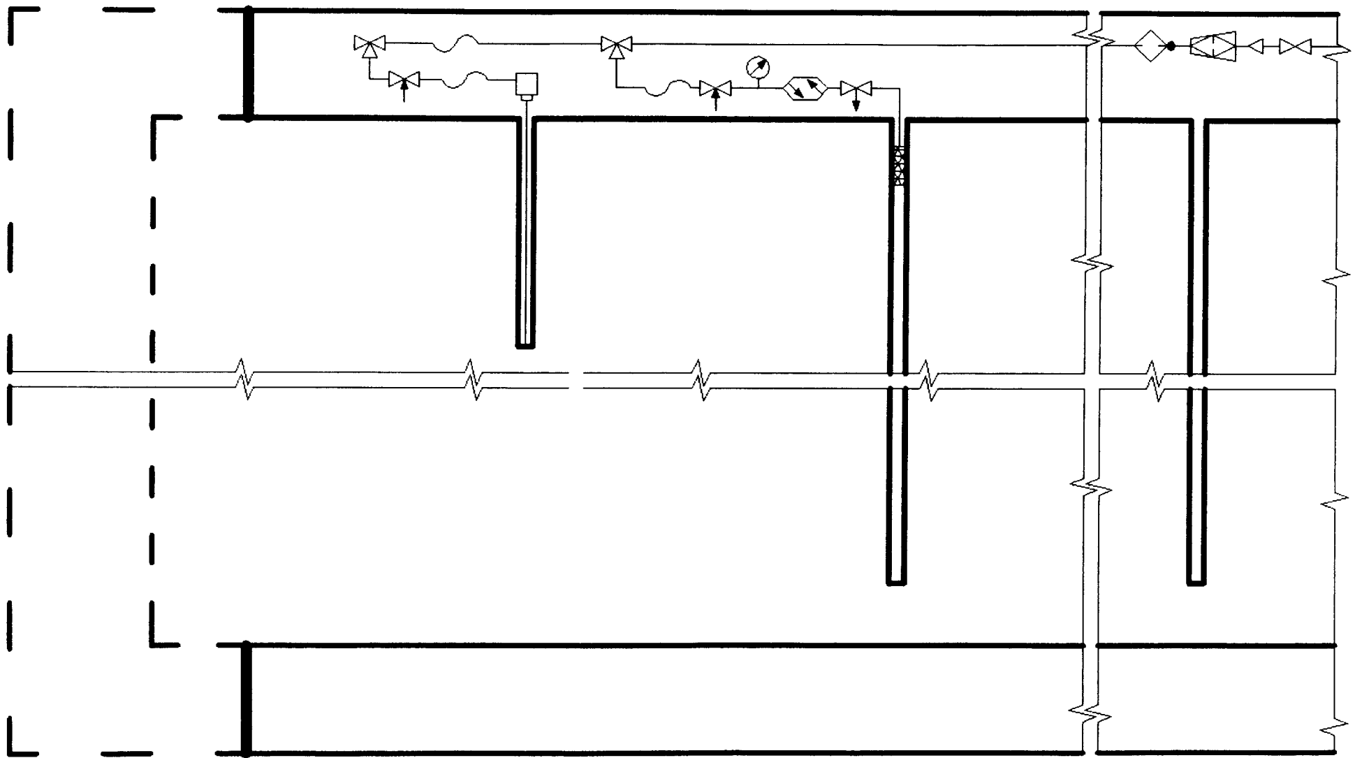
Рис. 6. Технологическая схема предварительного нагнетания жидкости в пласт из противопожарно-оросительного трубопровода через скважины, пробуренные из одной подготовительной горной выработки (схема б)
