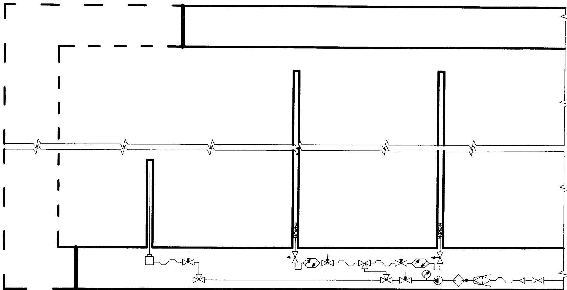
Рис. 8. Технологическая схема увлажнения очистного блока по мере его подготовки в режиме высоконапорного нагнетания жидкости насосной установкой. Бурение скважин с вентиляционного или конвейерного штрека (схема 8)
