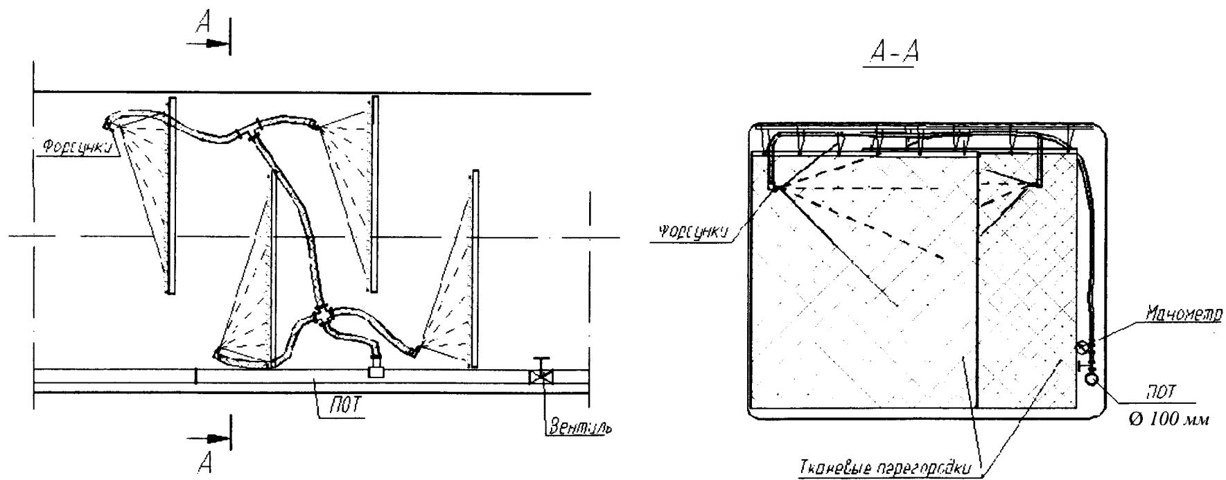
Рис. 1. Схема установки лабиринтной завесы
