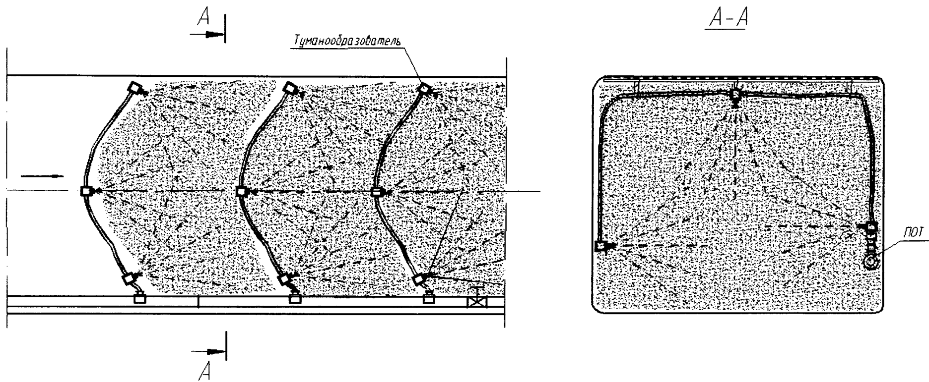
Рис. 2. Схема установки туманообразующих завес
