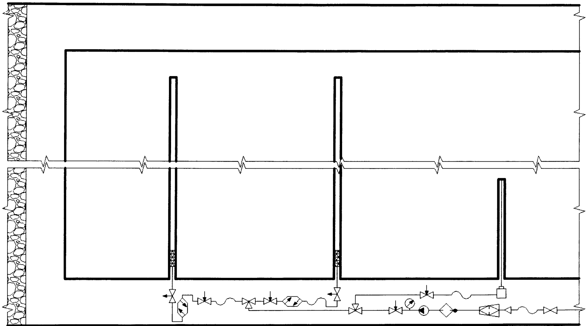
Рис. 1. Технологическая схема нагнетания жидкости в угольный пласт насосной установкой через скважины, пробуренные из подготовительной горной выработки (схема 1)
