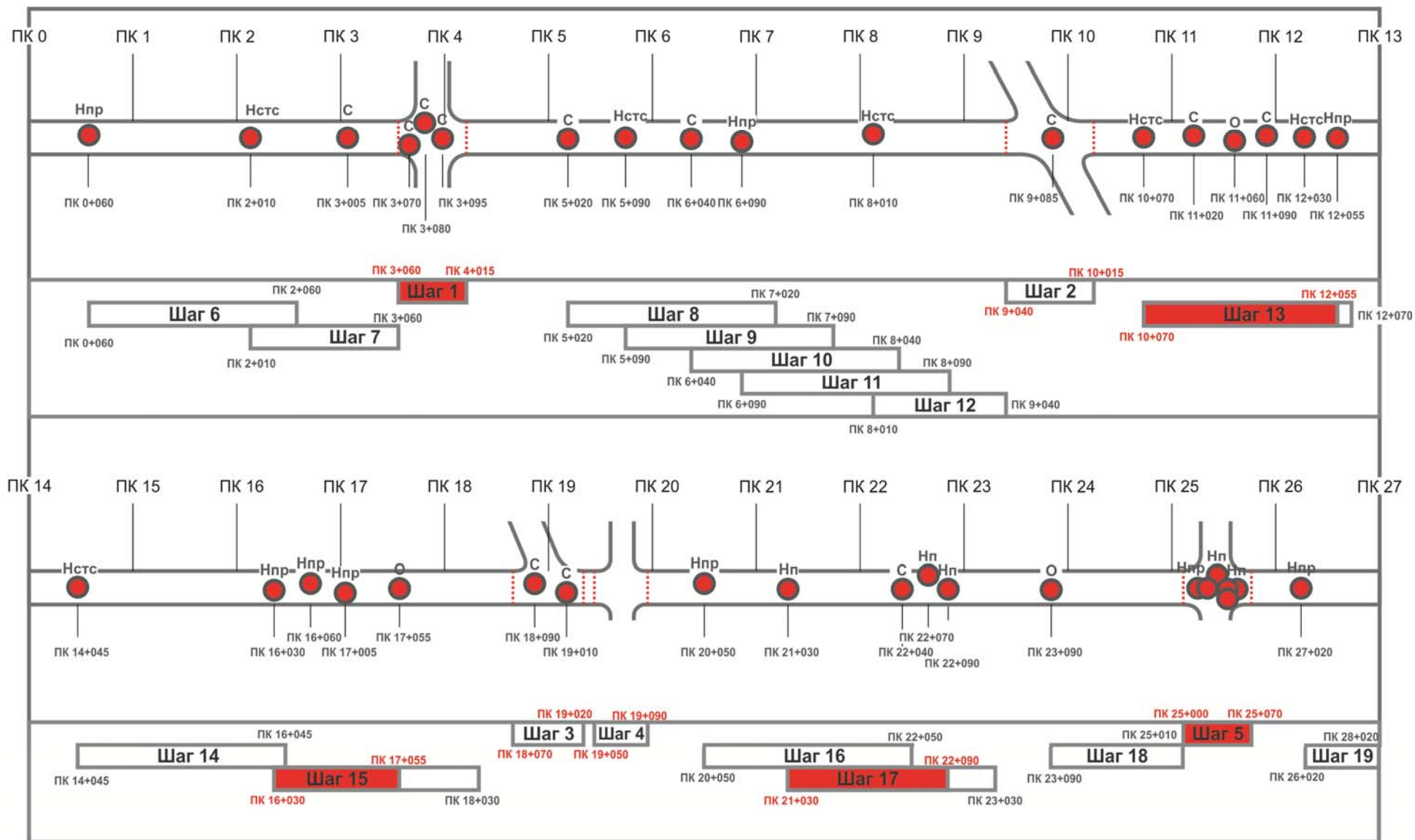
Рисунок Е.2 – Пример выявления мест концентрации ДТП на участке дороги в пределах населенного пункта
